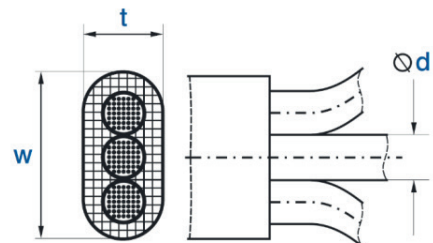
Kablo Ölçüleri/Cable Dimension
